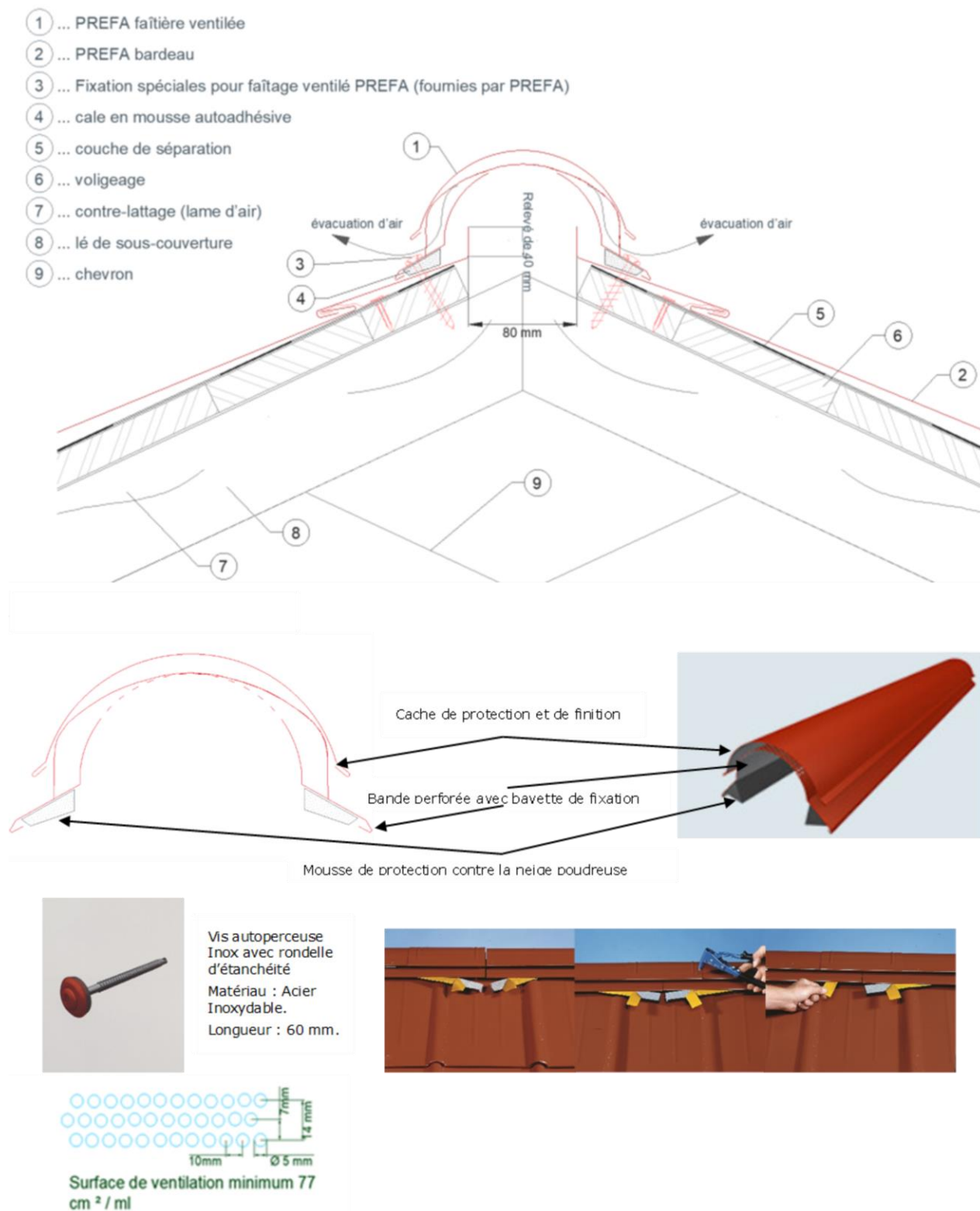
Figure 12.2- Faîtage ventilé PREFA – Climat de plaine (S= 150 cm 2 /ml)
