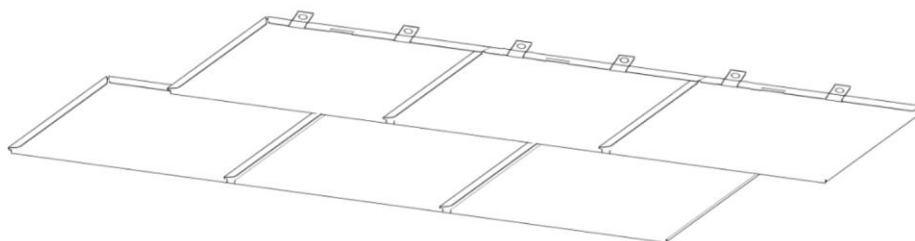
Figure 10 – Emplacement des pattes de fixation en zone d'angle de toiture (cf. figure 11) : 2 pattes par Bardeau
