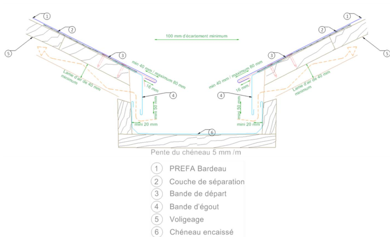
Figure 16– Chéneaux (climat de plaine)
