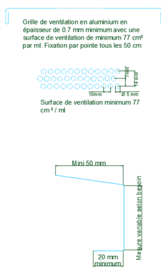
Figure 12.3 - Ventilation de la faîtière en climat de montagne
