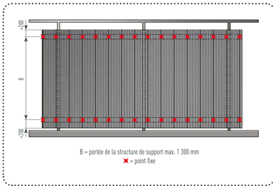
Figure 7 · Profil triangle monté à la verticale
