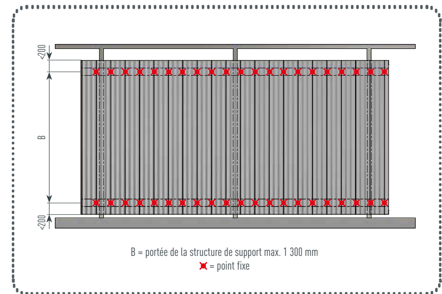
Figure 5 · Profil sinus monté à la verticale
